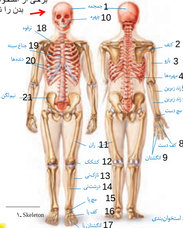
شکل ۷- دستگاه حرکتی
