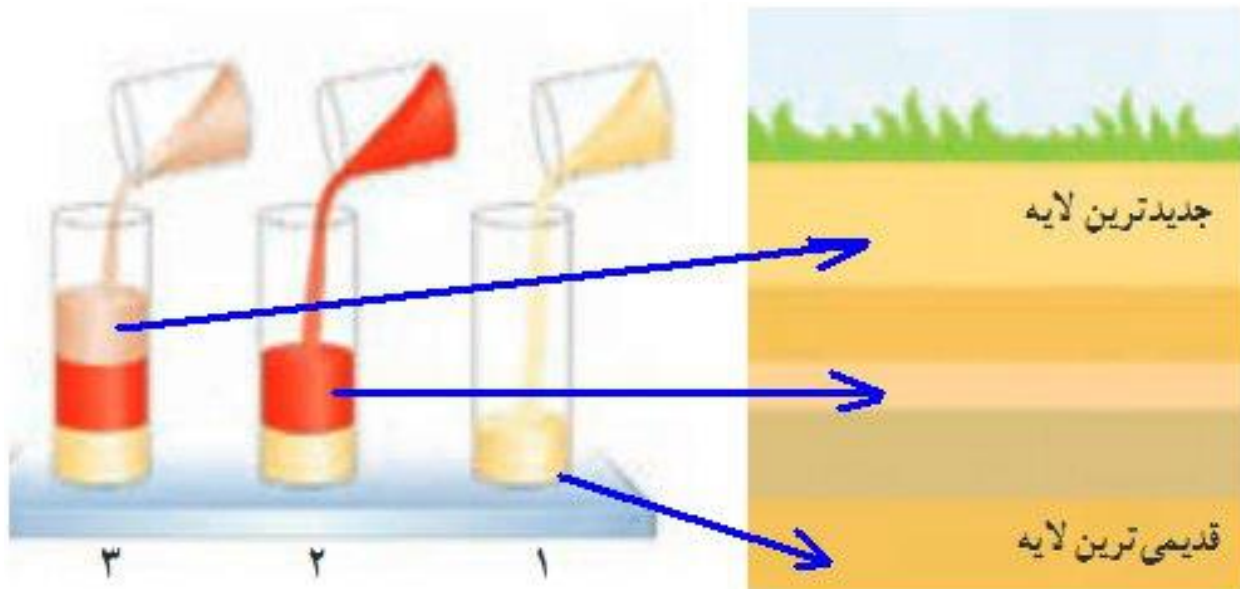
شکل ۱۳- نحوه تشکیل توالی از لایه‌های رسوبی
